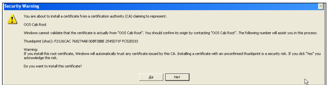
Рис. 39 Подтверждение импорта
