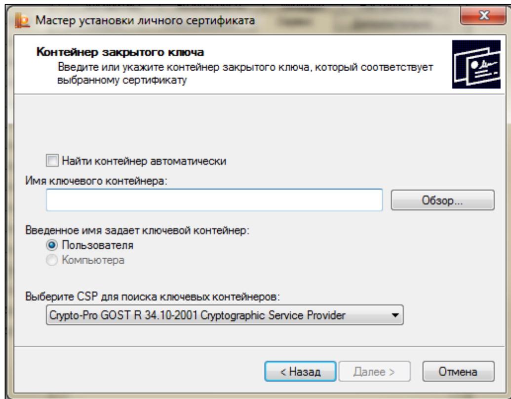
Рис. 61 Выбор контейнера
