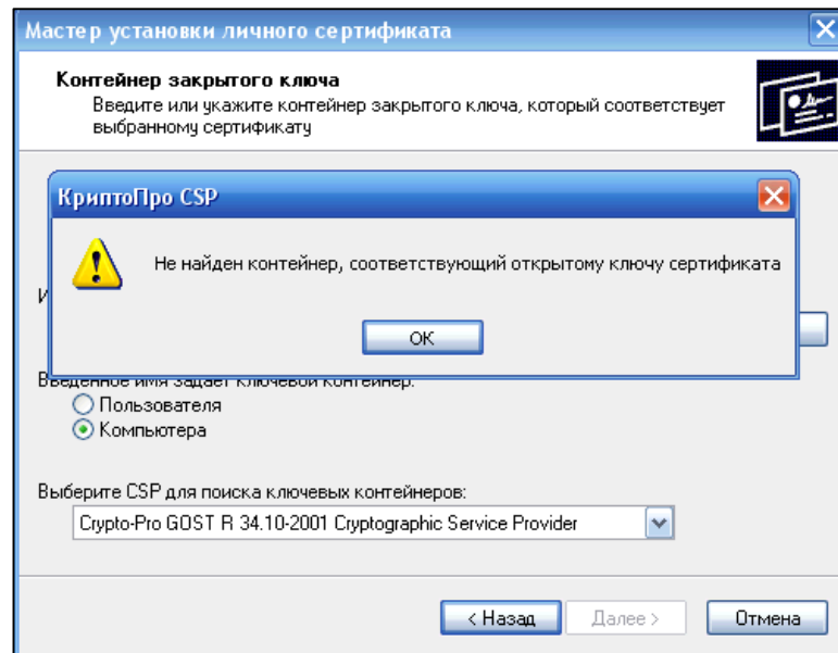
Рис. 79 Отсутствует контейнер
